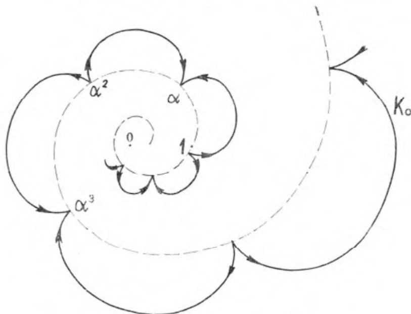
Hüllbahn einer eingliedrigen Kette (Nullstelle \zeta_k einfach)
